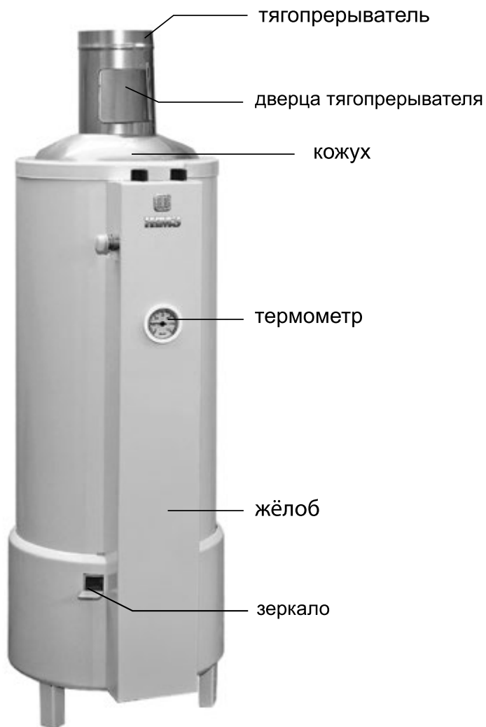
Рисунок 8. Аппарат Комфорт
